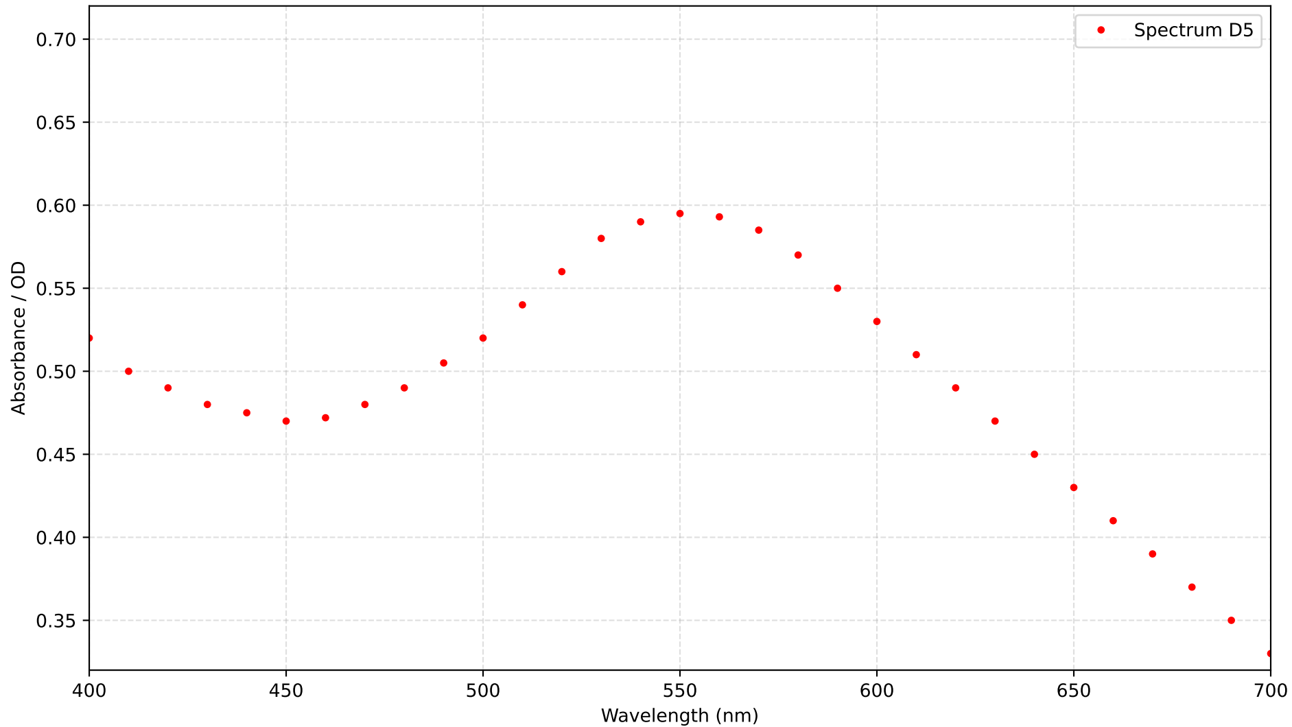
Spectrum - D5
